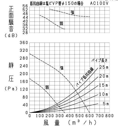
VD-23ZB 13 -IN/P-Q・騒音特性
